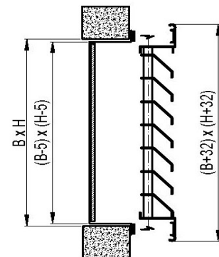
GR22: fissaggio con magneti
