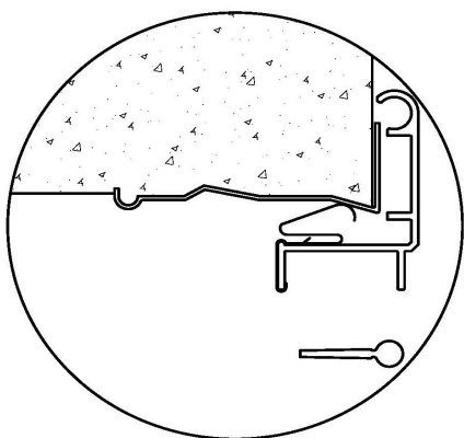
Montaggio con bocchetta a singola deflessione
