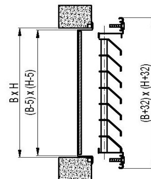
GR23: fissaggio con viti
