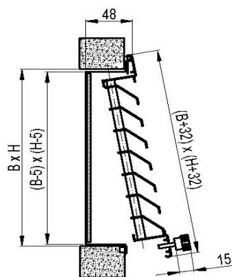
GR4: fissaggio con pomelli
