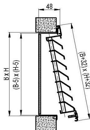
GR3: fissaggio con viti
