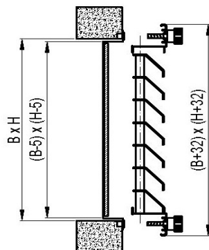
GR24: fissaggio con pomelli
